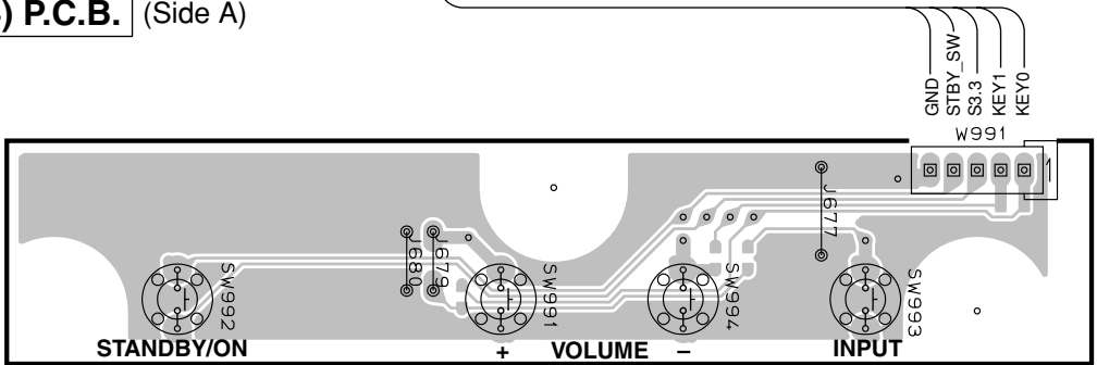
INPUT (4) P.C.B. (Side A)
